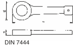
DIN 7444
